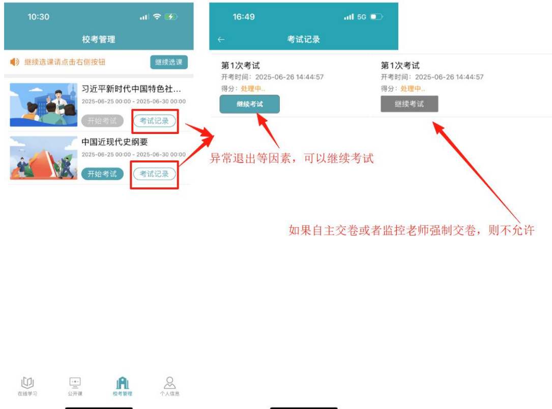
(图 - 异常处理)
